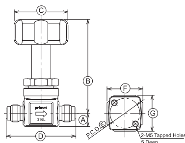
Male Metal Seal メタルシールオス
